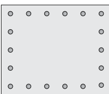
MH08.O 1020x840x65mm
